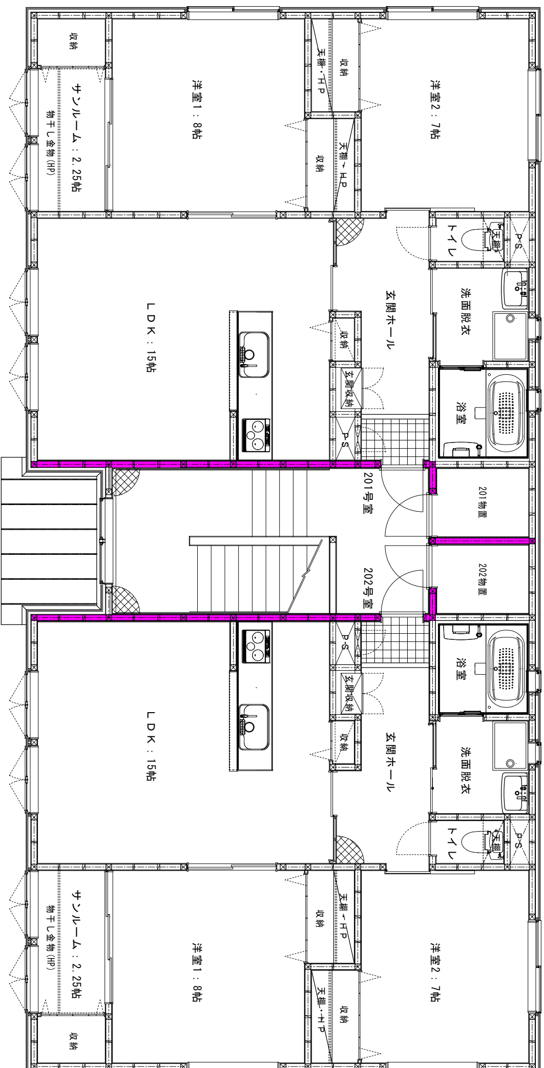
2階平面図
