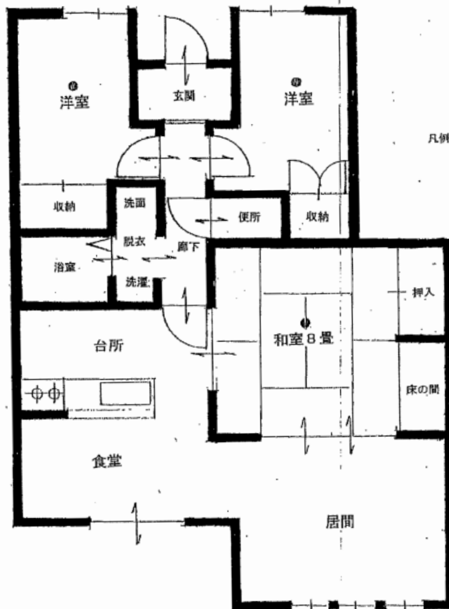
住戸平面図 火災警報器配置図) S=1:50
